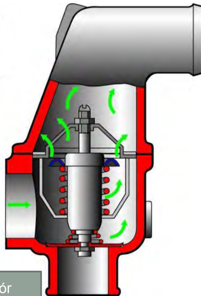
Termostat otwarty
