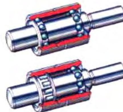
Trzpień obrotowy z dwoma łożyskami kulkowymi (u góry) i z łożyskiem kulkowym oraz wałeczkowym (u dołu)
