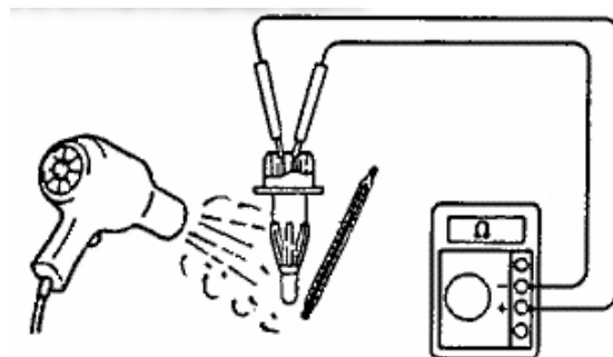
Sprawdzanie czujnika temperatury cieczy chłodzącej
