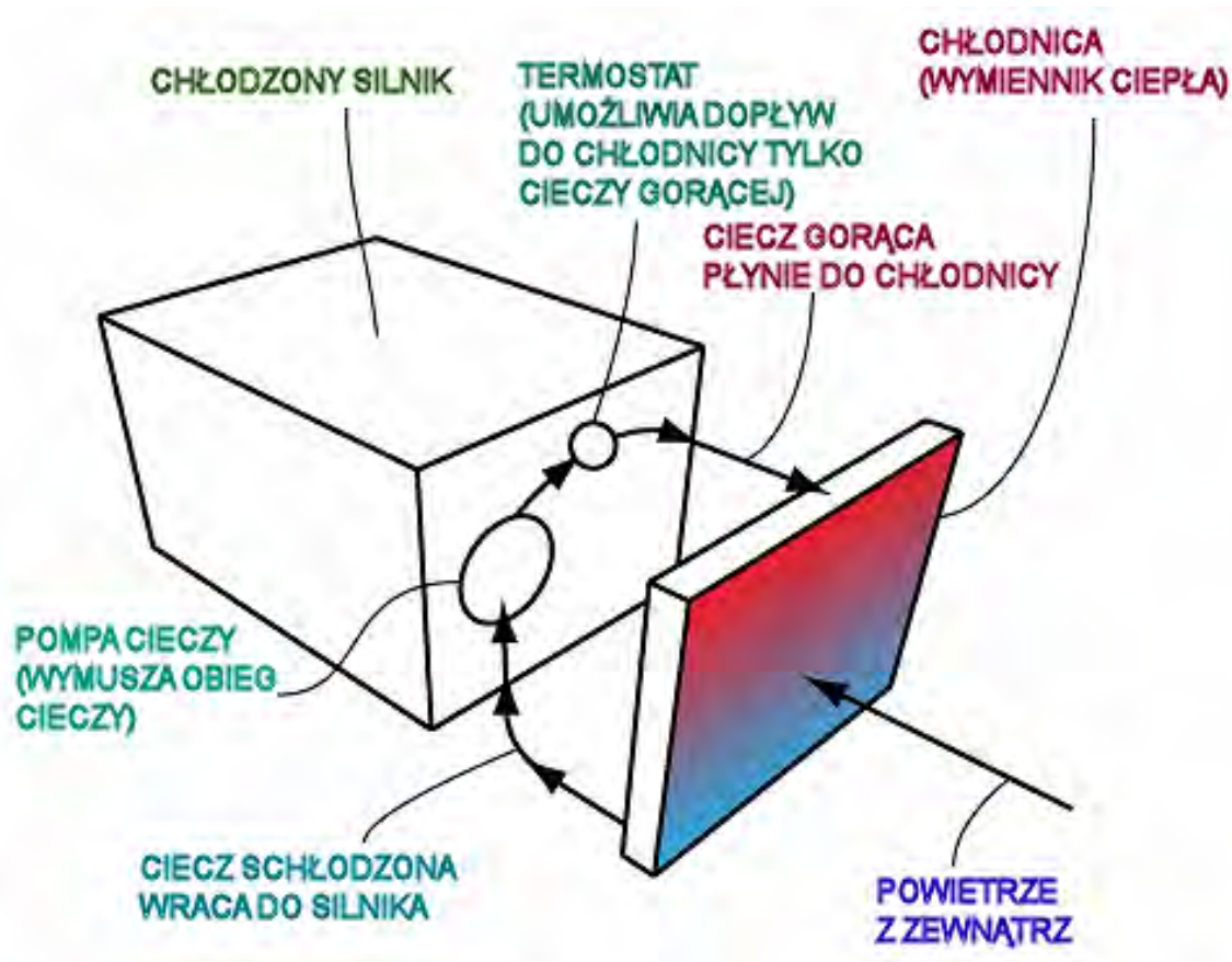
Schemat ideowy układu chłodzenia pośredniego silnika spalinowego
