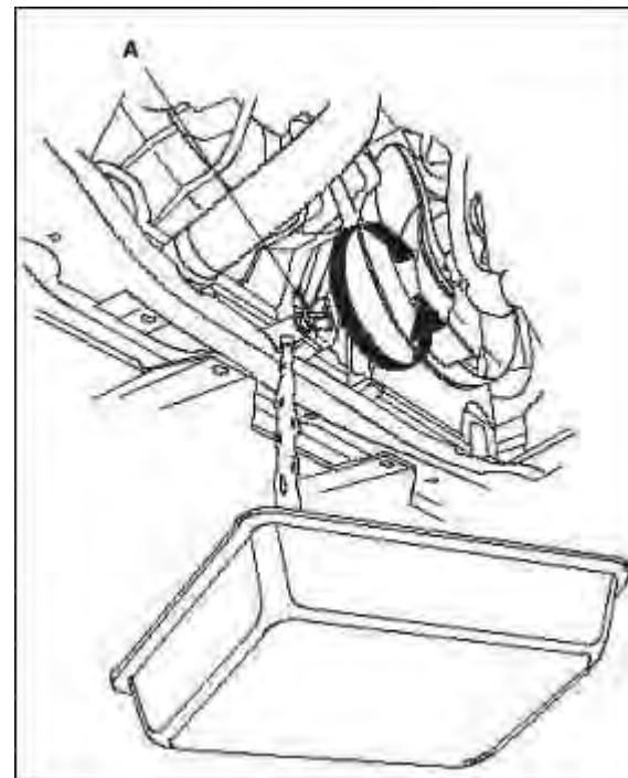
A- zawór spustowy chłodnicy
