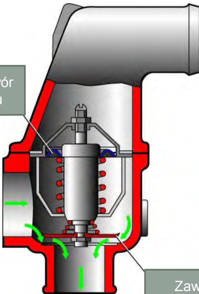
Termostat zamknięty
